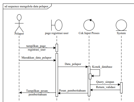
Gambar, 5 Sequence Diagram dari Mengelola Data Pelapor
