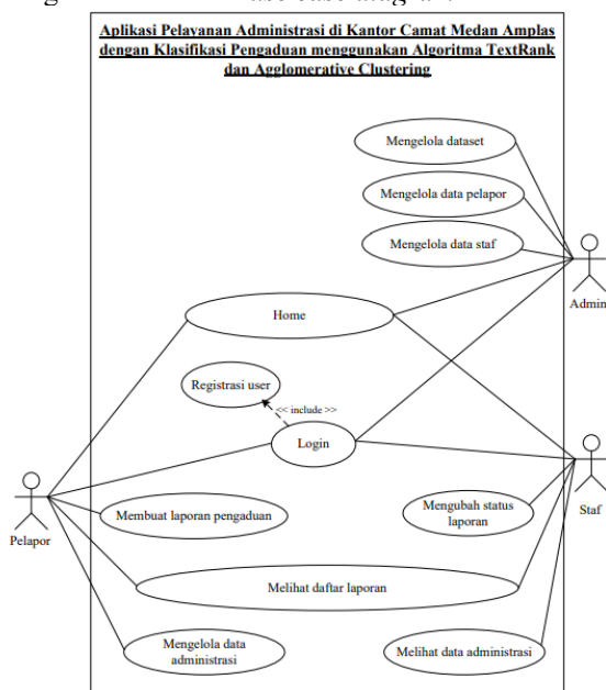
Gambar. 4 Use Case dari Aplikasi Pelayanan Administrasi
