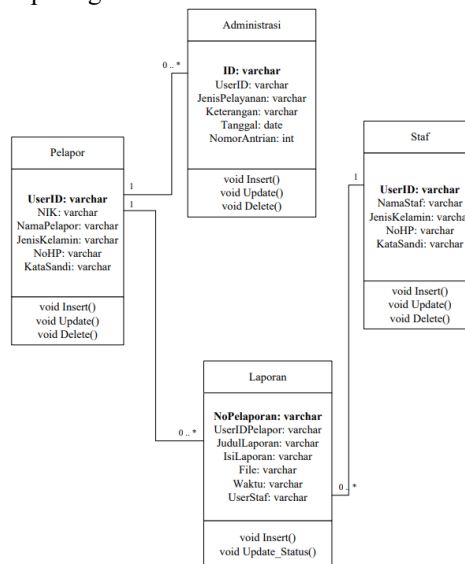
Gambar. 6 Class Diagram dari Aplikasi Pelayanan Administrasi di Kantor Camat Medan Amplas
