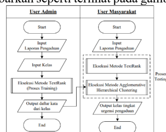
Gambar 2. Flowmap dari Aplikasi Pelayanan Administrasi
