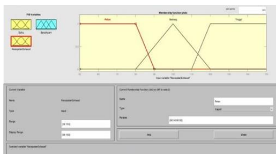
Gambar. 3 Kecepatan Exhaust Berdasarkan Tingkat Kelembapan
