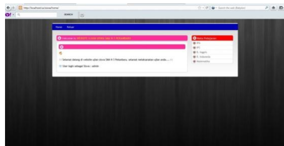
Gambar 2. Menu Utama
