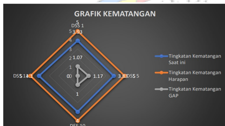
Gambar 3. Grafik kematangan
