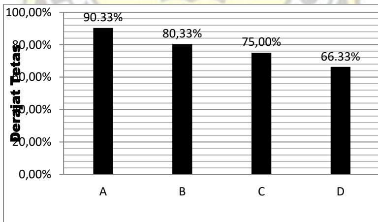
Gambar 1. Histogram Derajat Penetasan Telur Ikan Patin
