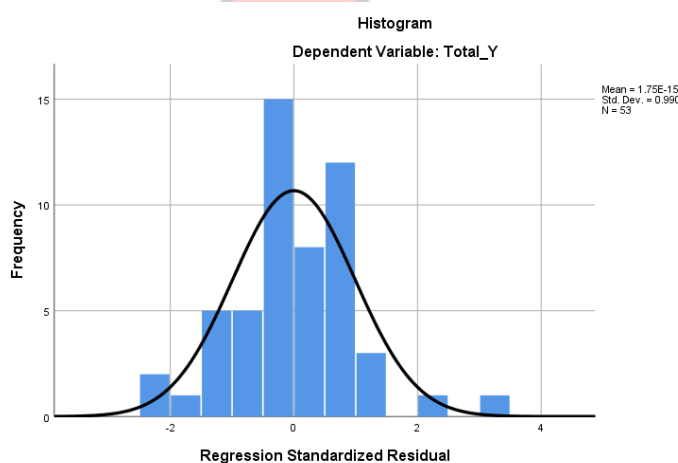
Gambar 4.10 Grafik Histogram
