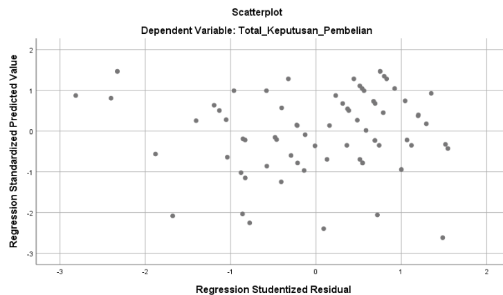
Gambar 2 Pengujian Heteroskedastisitas
