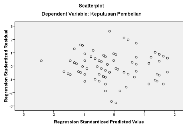
Gambar Hasil Uji Heterokedastisitas (Scatterplot)
