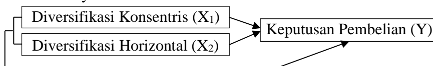
Gambar Kerangka Pemikiran
