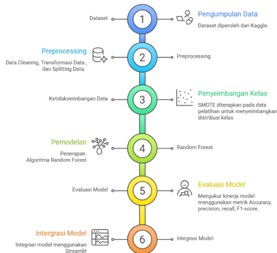
Gambar 1. Tahapan Penelitian
