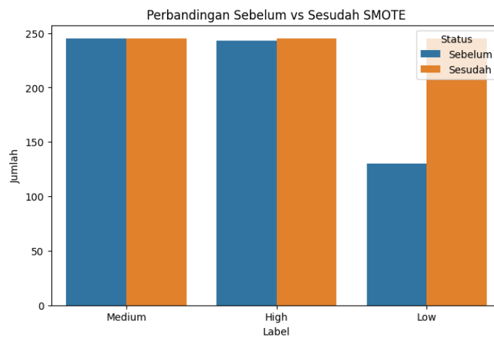
Gambar 2. Hasil Perbandingan SMOTE
