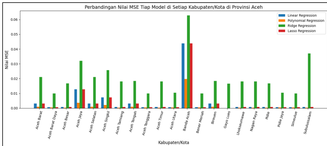
Gambar 2. Perbandingan Nilai MSE Tiap Model
