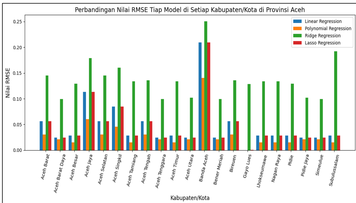
Gambar 1. Perbandingan Nilai RMSE Tiap Model
