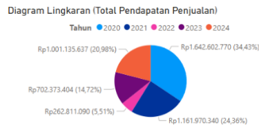
Gambar 7 Diagram Lingkaran
