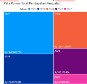
Gambar 6 Peta Pohon
