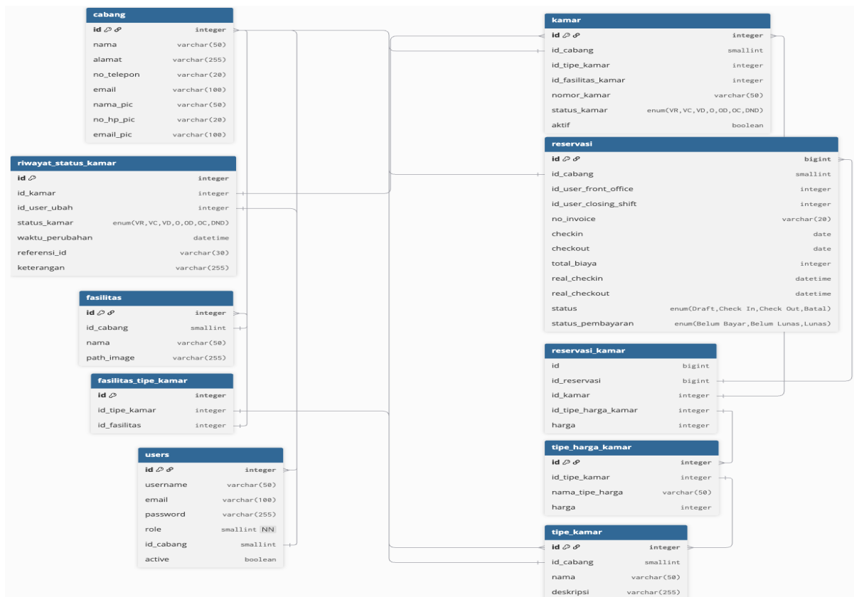
Gambar 9. Entity Relationship Diagram (ERD) Sistem Informasi Manajemen Hotel Multi-Cabang
