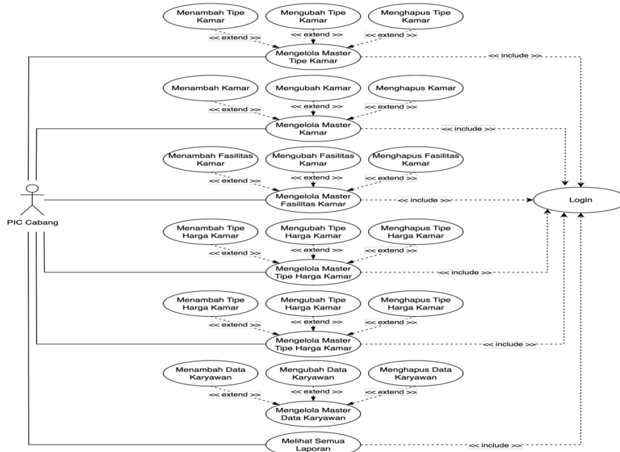
Gambar 3. Use Case Diagram Aktor PIC Cabang
