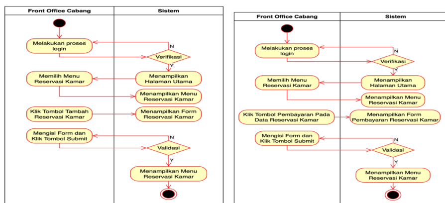
Gambar 7. Activity Diagram Menambah Reservasi Kamar dan Pembayaran Reservasi Kamar (Dari Kiri)
