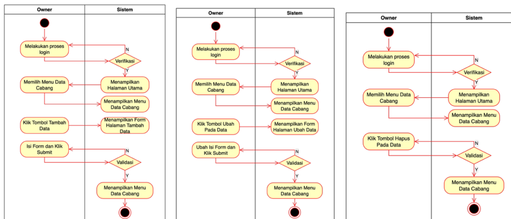
Gambar 6. Activity Diagram Mengelola Master Data Cabang (Dari Kiri)
