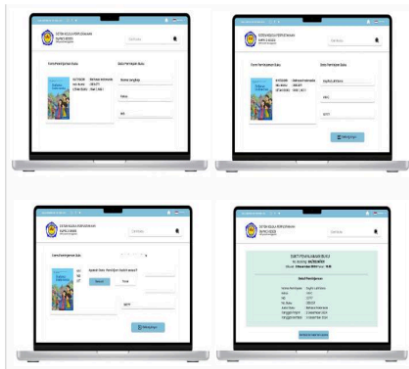
Gambar 9.Design Alur Peminjaman Buku
