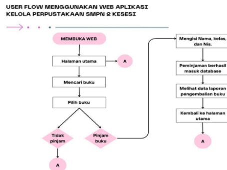
Gambar 5. User Flow Web Aplikasi Kelola Perpus
