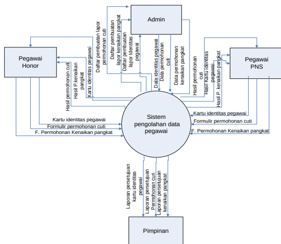
Gambar 1. Diagram Konteks Pengolahan Data Pegawai
