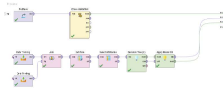
Gambar 3. Proses Data Mining dengan Metode Decision Tree dan Validasi Silang
