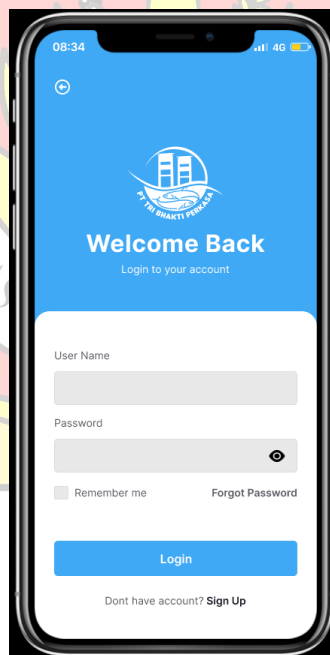
Gambar 2. Halaman Login
