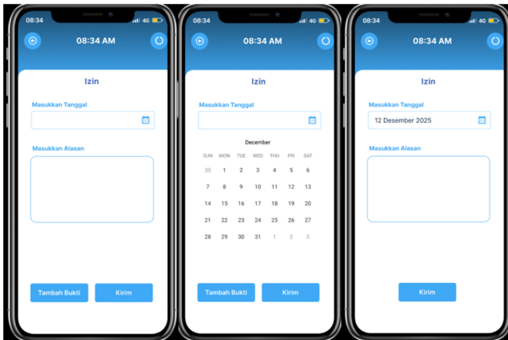
Gambar 6. Halaman Izin
