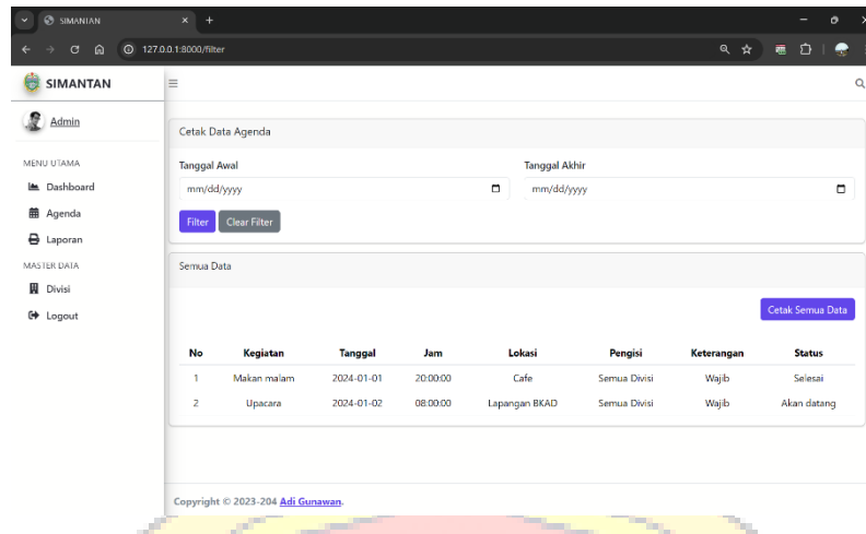
Gambar 10. Halaman Laporan
