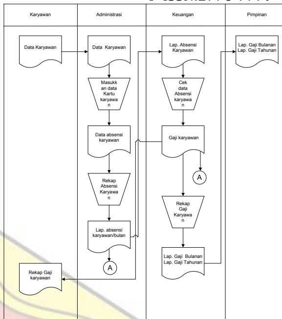
Gambar 1. Flow Map PT. Semen Andalas yang sedang berjalan
