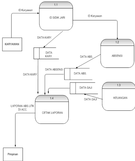
Gambar 2. DFD Level 1 Sistem Informasi Absensi
