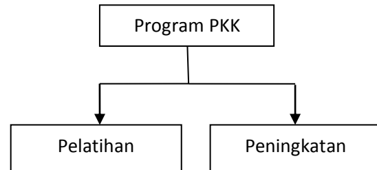
Gambar 1. Kerangka Teoritis
