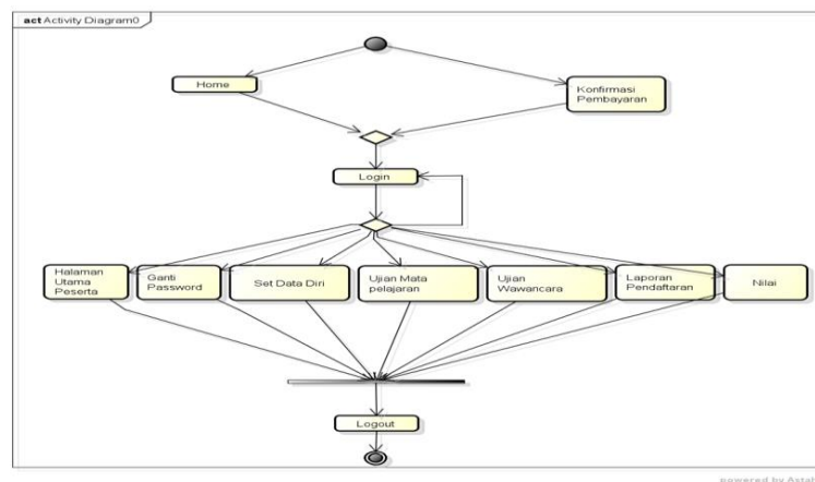
Gambar 2 Activity Diagram Calon Peserta Didik Baru
