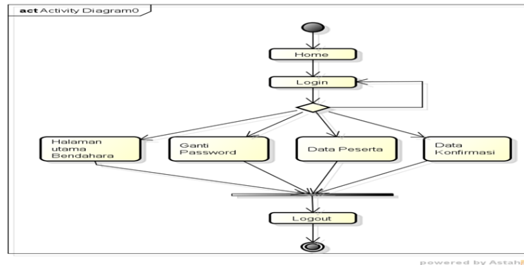
Gambar 3 Activity Diagram Bagian Keuangan
