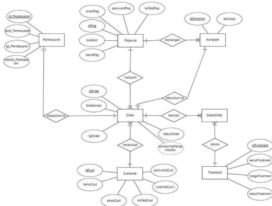
Gambar 4 ERD dari sistem informasi laundry sepatu XYZ
