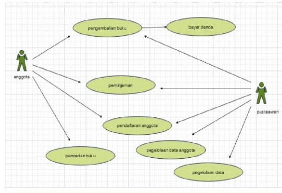
Gambar 1. Diagram Use Case yang sedang berjalan
