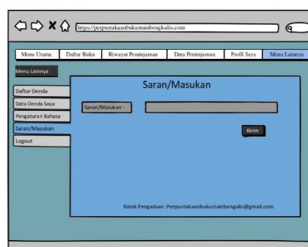
Gambar 12.1 Halaman Saran/Masukan
